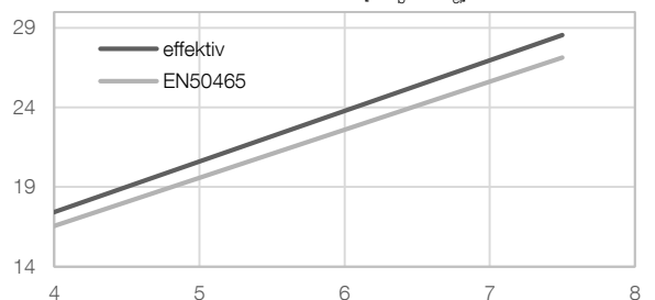
Verbrauchsskurven 2) [kW b / kW el ]
